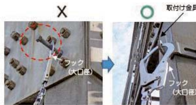
取付設備へのフックの掛け方(例)
